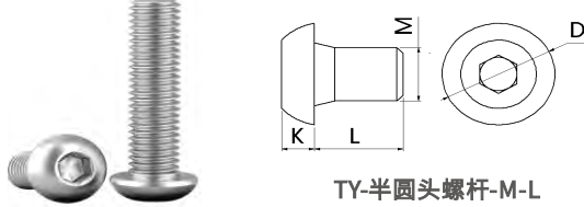
TY-半圆头螺杆-M-L
