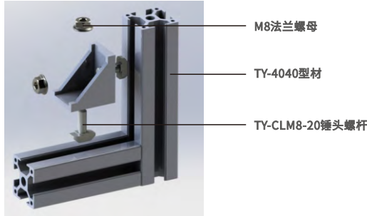
组装图
