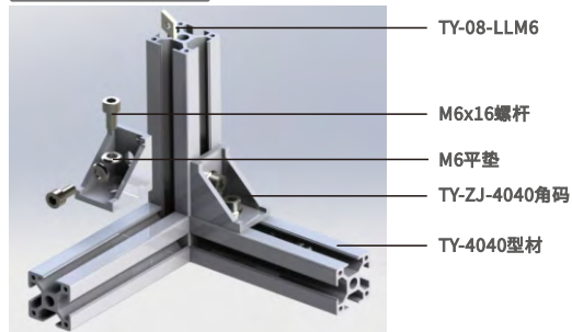
组装图
