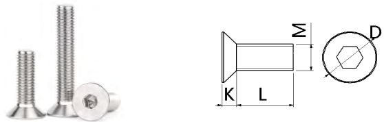
TY-平头内六角螺杆-M-L
